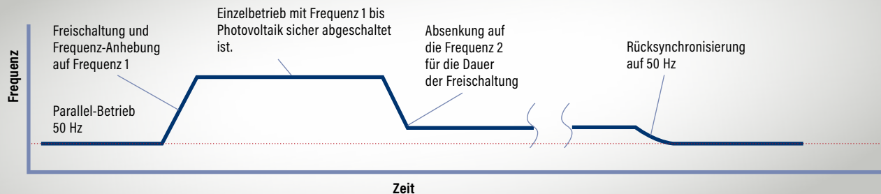
Schematischer Ablauf 50Hz Plus Betrieb
